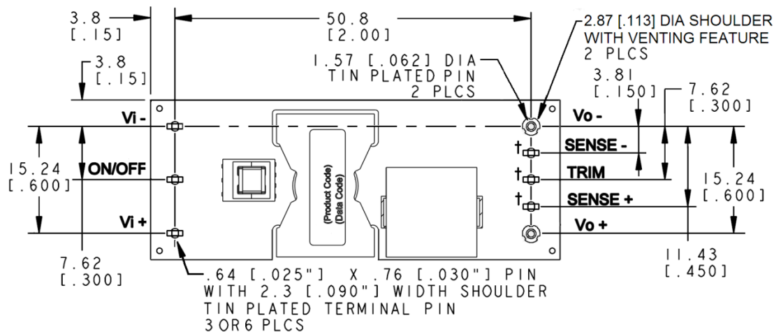
Bottom View*
