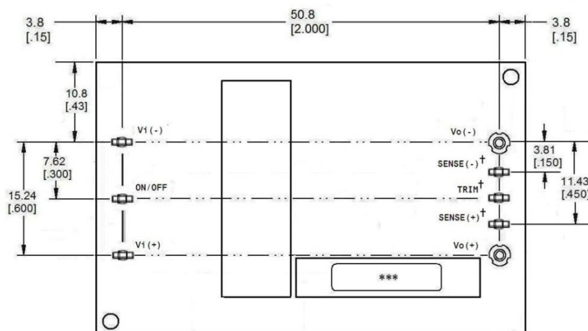
BOTTOM VIEW***
